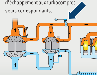
Suralimentation séquentielle (vue schématique)
