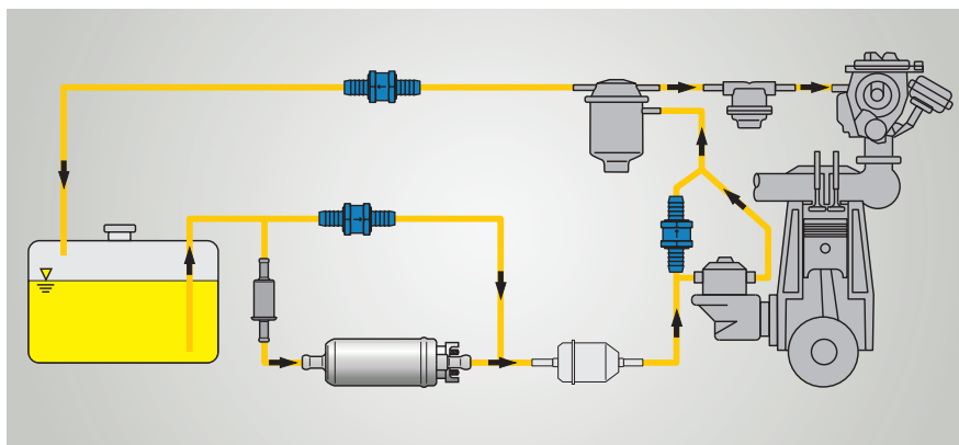
Exemple d'application : moteur à carburateur avec pompe supplémentaire électrique connectable
