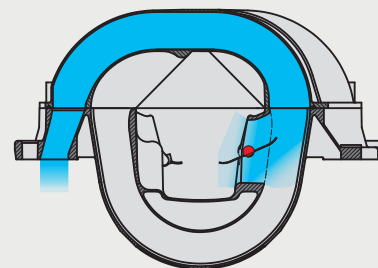
Clapet ouvert n > 3500 tours/minute l = 450 mm
