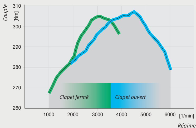
Clapet fermé n < 3500 tours/minute l = 890 mm
