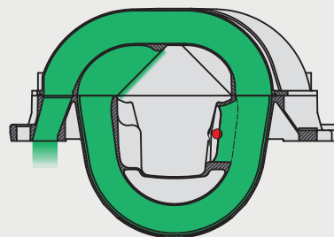
Clapet fermé n < 3500 tours/minute l = 890 mm
