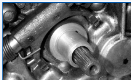
Desgaste del cojinete del árbol principal (movimiento)
