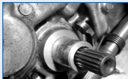
Desgaste del tubo guía de la transmisión.
