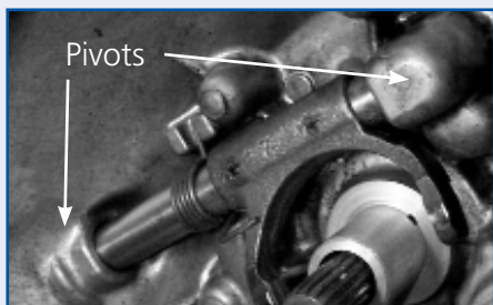
Un mecanismo de embrague gastado o agarrotado
