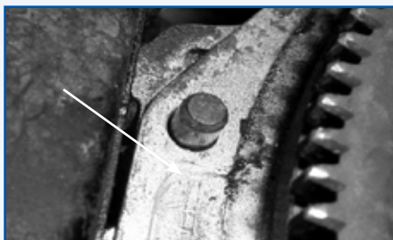
centradoras de la caja de cambios (faltan o dañadas)
