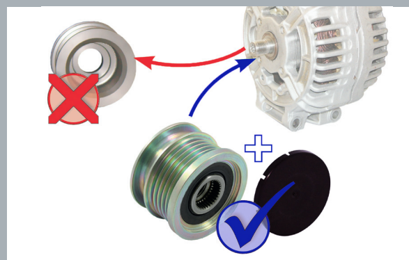
Figura 1: Cambio de polea rígida a una polea libre de alternador
