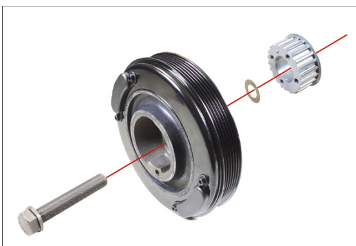
Fig. 1: Polea damper del cigüeñal con tornillo central del cigüeñal y arandela con recubrimiento de diamante
