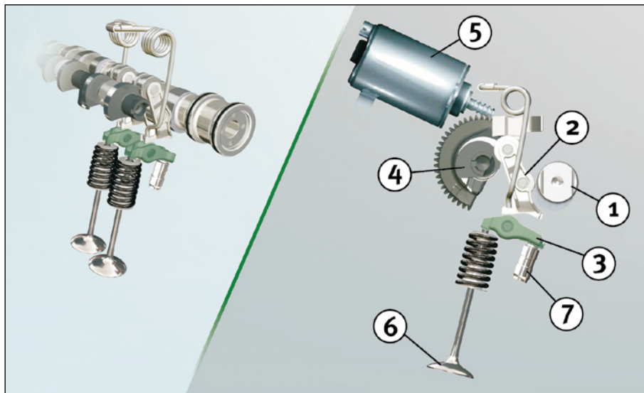
Image 1: vue d'ensemble du système du moteur Valvetronic de BMW/vue détaillée des composants du système
