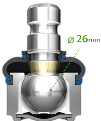
Diámetro ampliado de las bolas en la rótula
