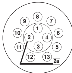
Kontaktbelegung 13 pol. der Steckdose
