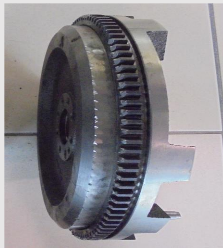
Ci contre le volant moteur du kit 835053 avec la couronne positionnée au centre. On note ici suite à une mauvaise affectation que les dents du démarreur ont usiné celles de la couronne du volant moteur.
